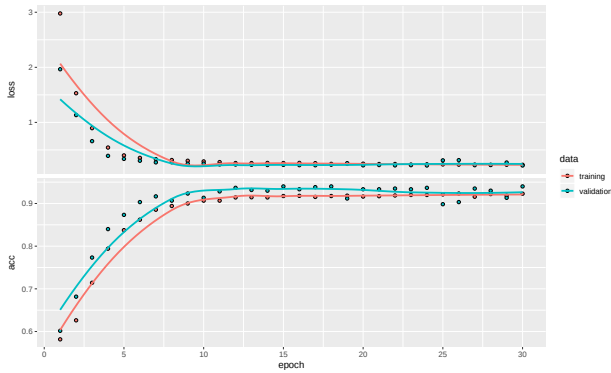
FIGURE 10.14 – Evolution des erreurs en fonction de l'epochs.
