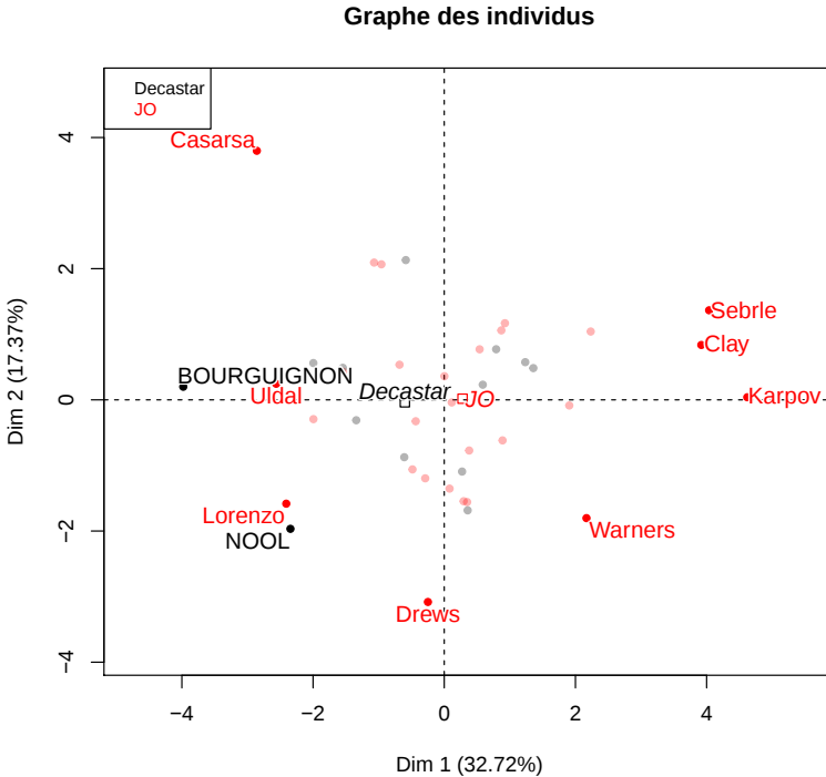
FIGURE 7.3 – ACP sur le décathlon : graphe des individus.
