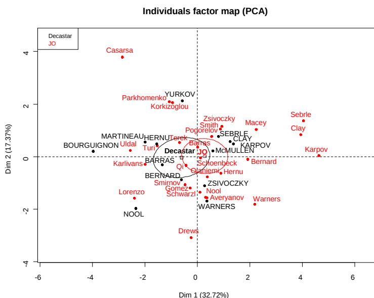
FIGURE 7.4 – Ellipses de confiance autour des modalités d’une variable qualitative.
