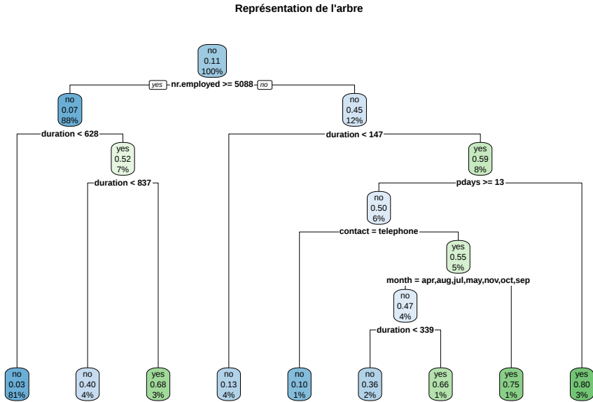
FIGURE 9.14 – Arbre de classification : prédire la variable y.
