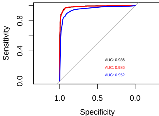
FIGURE 10.5 – Courbes ROC et AUC des forêts aléatoires avec mtry=7 (noir), mtry=10 (rouge) et d'un arbre de classification (bleu).
