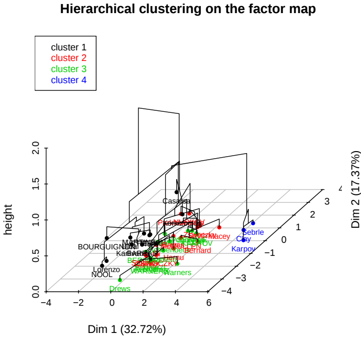
FIGURE 8.4 – Classification Ascendante Hiérarchique fournie par HCPC .
