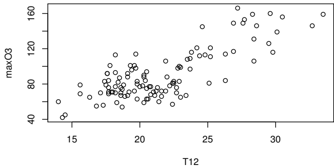
FIGURE 3.1 – Nuage de points (T12, maxO3) avec libellés des axes explicites.
