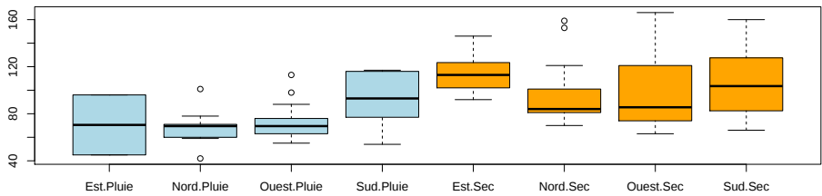
FIGURE 9.7 – Boîtes à moustaches du max03 selon le croisement des modalités de la variable vent et de la variable pluie.
