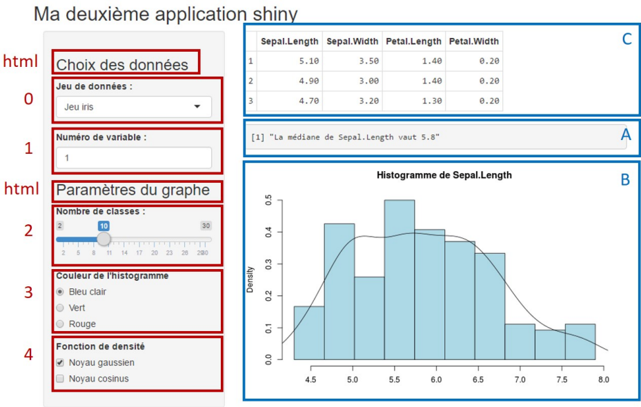
FIGURE 4.4 – Deuxième application shiny.
