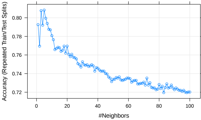
FIGURE 10.3 – Précision en fonction du nombre de plus proches voisins.
