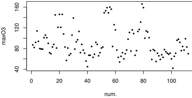
FIGURE 3.5 – Nuage de points des pics d’ozone ( maxO3 ) en fonction de l’index.
