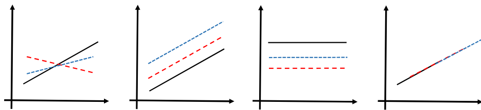
FIGURE 9.9 – Illustration des modèles d'analyse de covariance : représentation de Y en fonction de X , chaque modalité de Z est représentée par une couleur.
