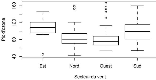
FIGURE 3.2 – Graphique avec plot des vecteurs vent et max03 .
