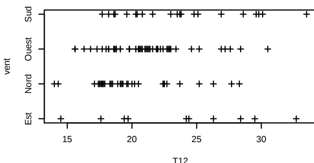
FIGURE 3.4 – Graphique d'une variable quantitative en abscisse ( T12 ) et d'une variable qualitative en ordonnée ( vent ).
